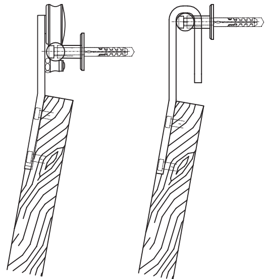
Rollwagen für Holzleiter Einhängelasche für Holzleiter Trolley for wooden ladders Hook bracket for wooden ladders
